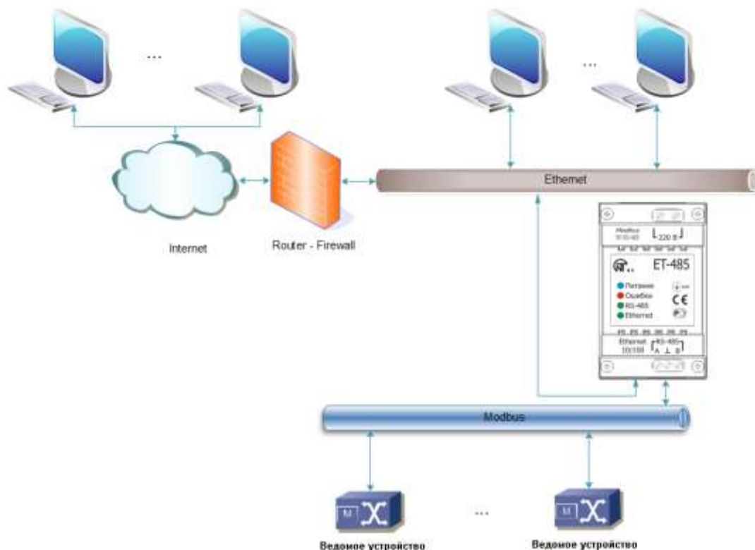
Рисунок Б.1 – Доступ к сети RS-485 (Modbus RTU/ASCII) по сети Ethernet (Modbus TCP)
