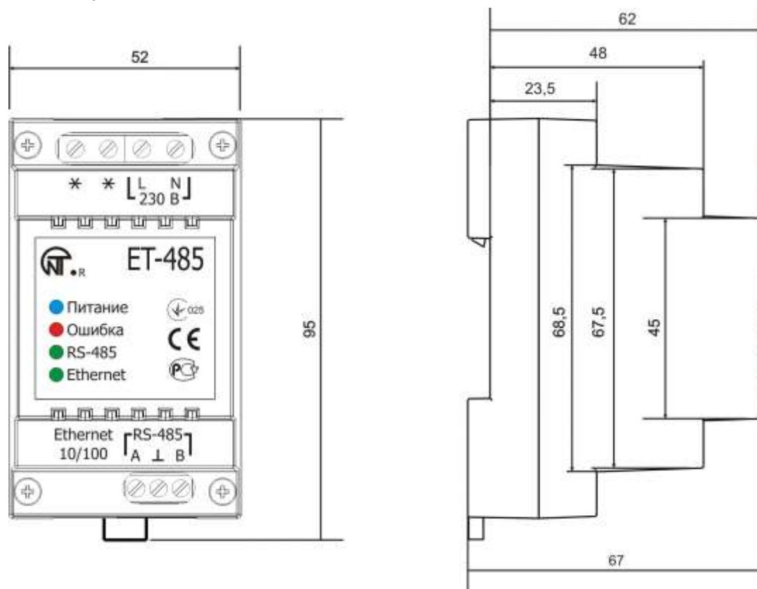
Рисунок 1 – Габаритные размеры прибора
