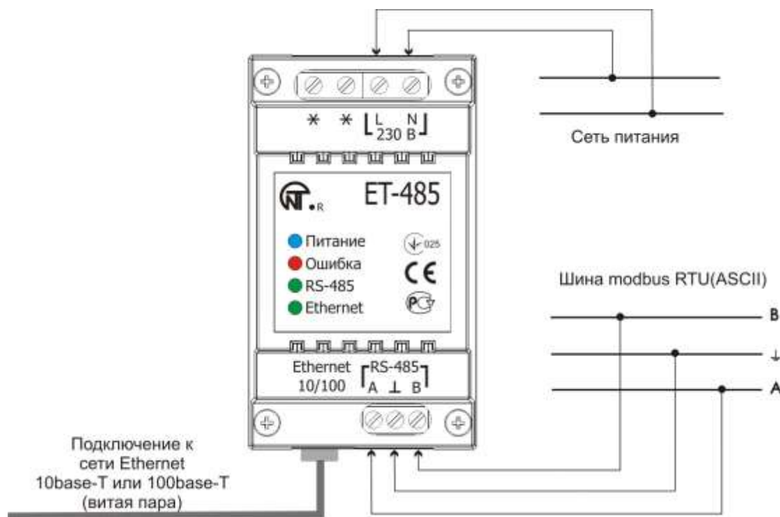
Рисунок 4 – Схема подключения прибора
