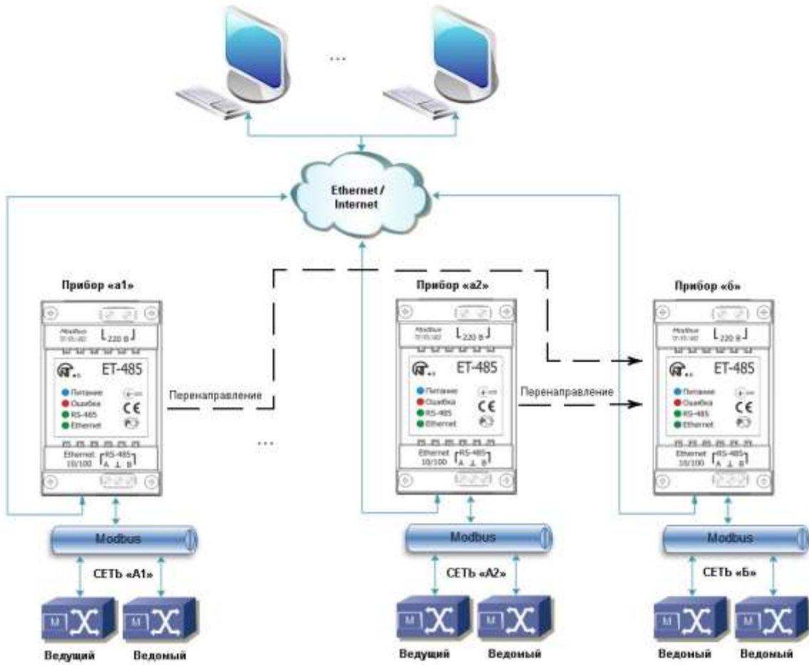
Рисунок Б.3 – Подключение двух независимых сетей Modbus к третьей сети
