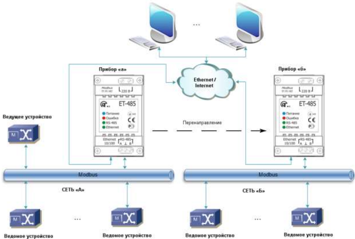
Рисунок Б.2 – Удлинение сети RS-485
